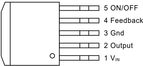
TO263-5L
