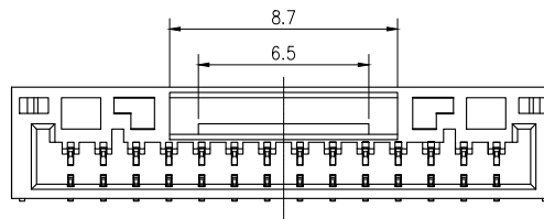
14PIN~16PIN
