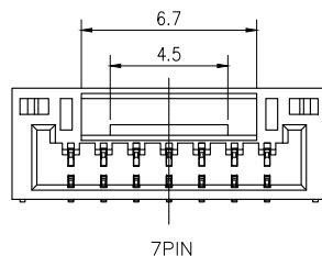
7PIN
